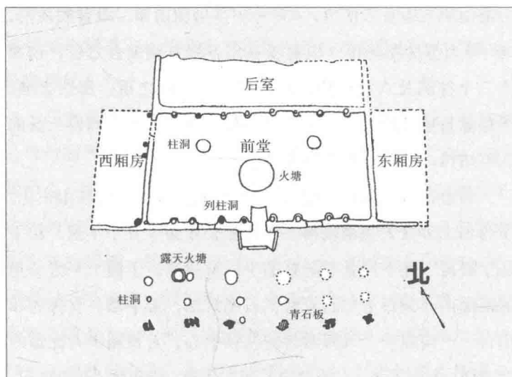
大地湾 901 号大型房址平面图
